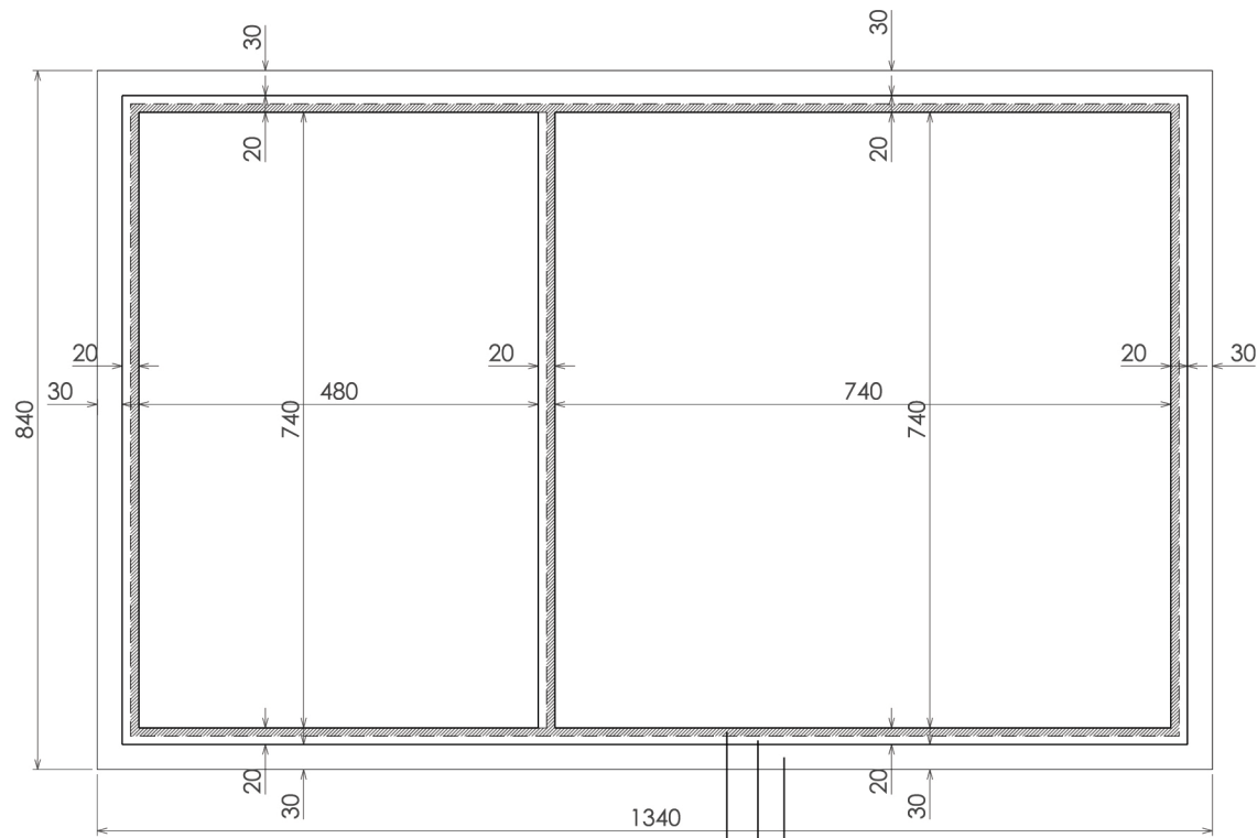
PIANTA FONDAZIONI - PLATEA
