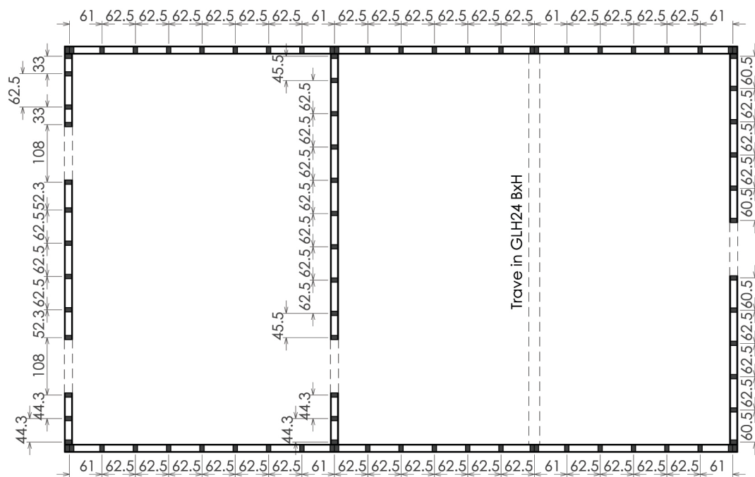
PIANTA ELEVAZIONI - PLATFORM FRAME
