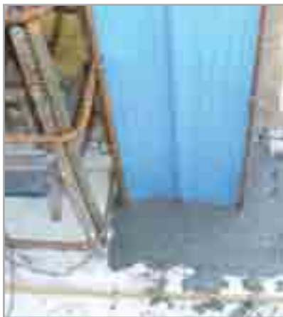
Fig. 7.56e - Ripristino della fondazione con MAPEGROUT COLABILE
