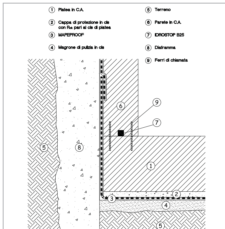
Fig. 7.40 - Particolare tecnico dell'applicazione di MAPEPROOF contro un diaframma reso collaborante alla struttura.
