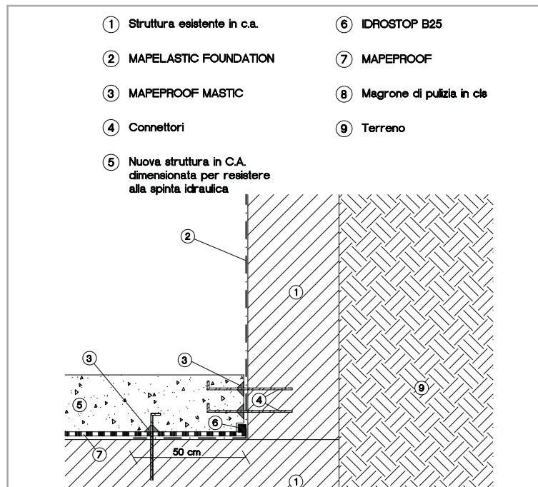
Fig. 8.7a - Particolare tecnico di una rifoderatura interna eseguita applicando MAPEPROOF sulla superficie orizzontale e MAPELASTIC FOUNDATION sulle verticali: raccordo tra soletta e parete controterra
