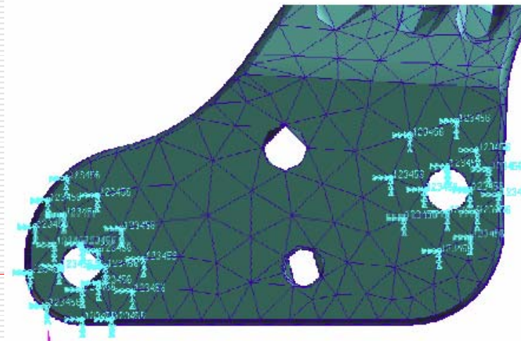
Figura 2 Particolare della Staffa Acqua-Mare
