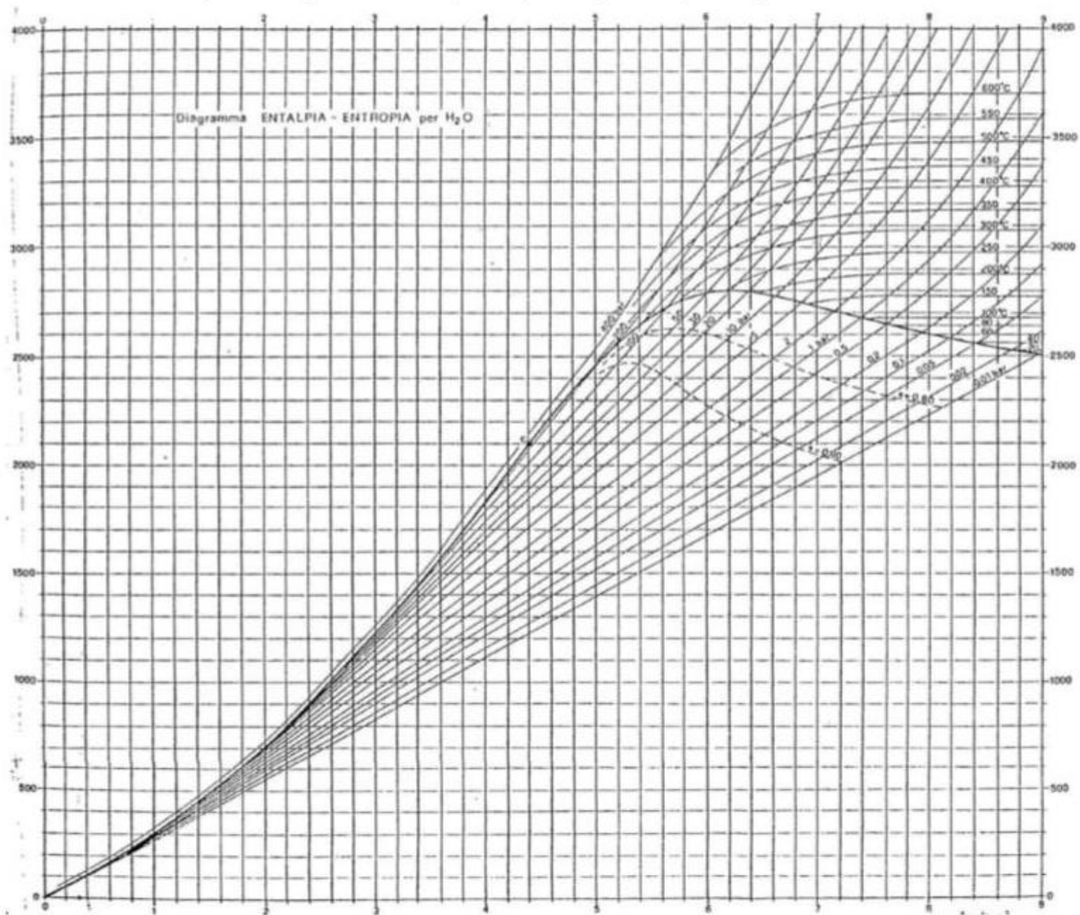
Figura 3 - Diagramma h-s dell'acqua: entalpia in \text{kJkg}^{-1} ed entropia in \text{kJkg}^{-1}\text{K}^{-1} .
