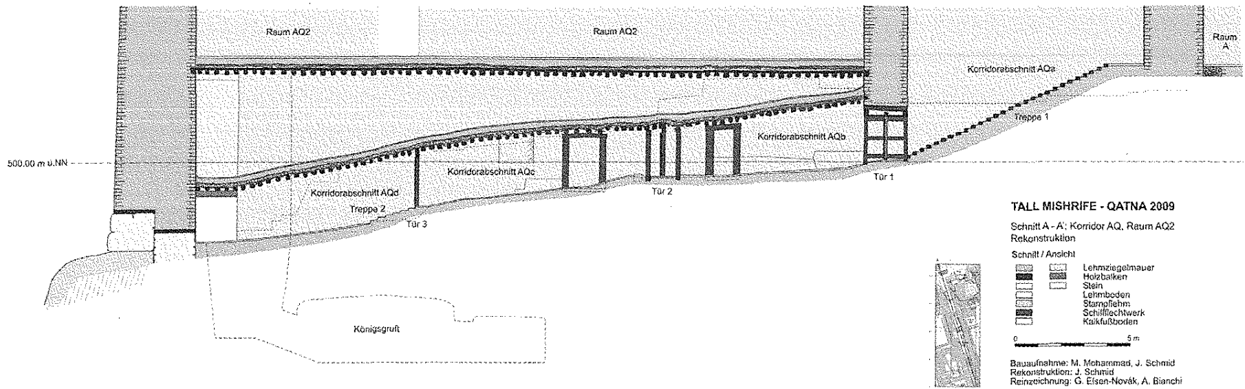
Abb. 17: Schnitt der Rekonstruktion des Korridors AQ und des darüberliegenden Raumes AQ 2 .
