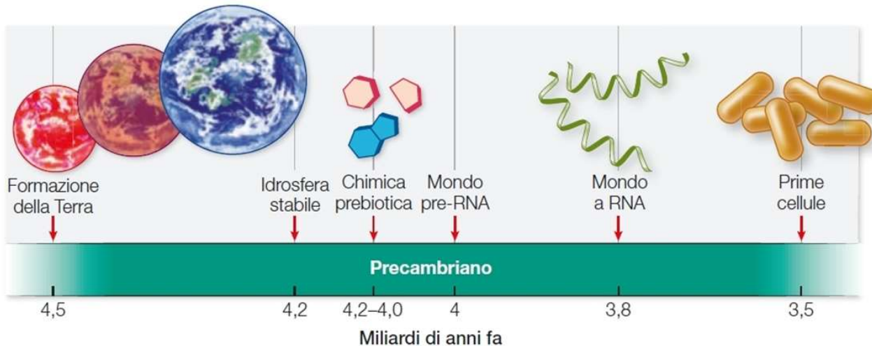
Figura 4.12 L'origine della vita Questa scala di tempi assai semplificata dà un'idea degli eventi principali culminati nell'origine della vita più di 3,5 miliardi di anni fa.
