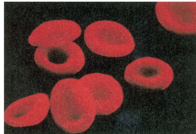
FIGURA I.11.1.2 Micrografia elettronica a scansione di eritrociti umani.
