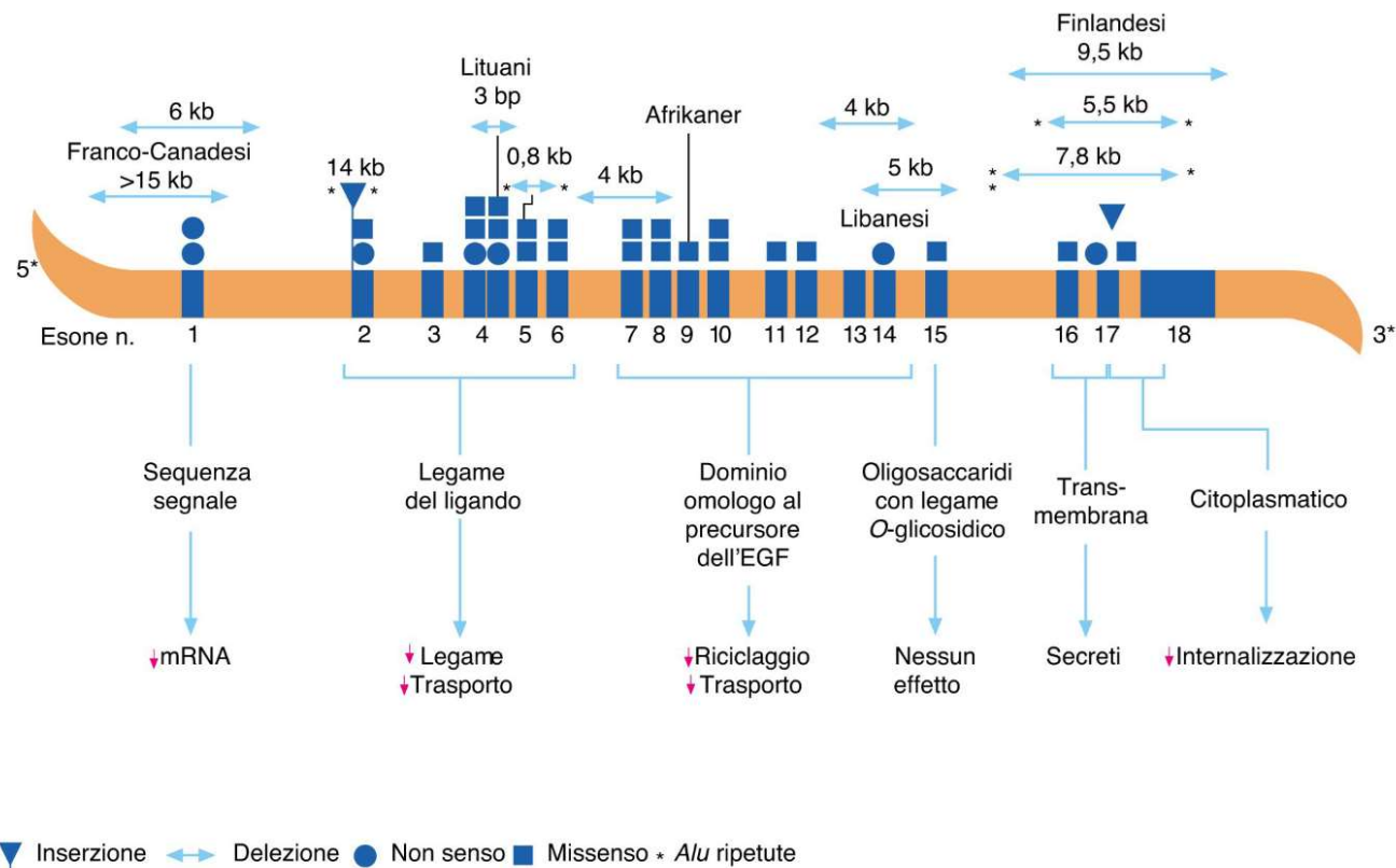
FIGURA 11.13 Gene del recettore LDL. Sono indicate le possibili numerose mutazioni puntiformi che lo interessano (nelle varie etnie) e le relative conseguenze fenotipiche e funzionali che causano la malattia.
