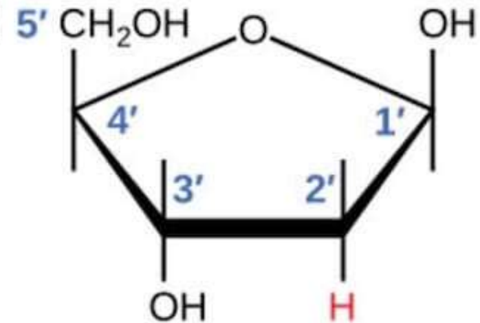
Desossiribosio
