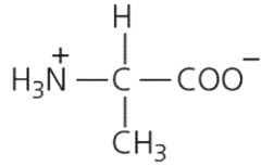
UN AMMINOACIDO
